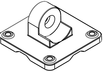
Sabit bağlantı elemanı Holding connection part قطعة التثبيت الثابتة
